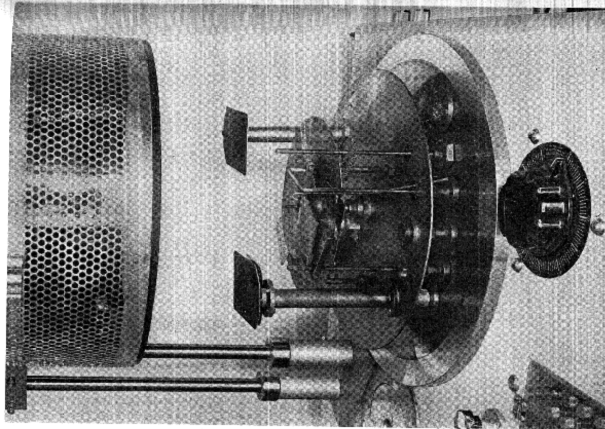
Fig. 14—Sputtering apparatus.
